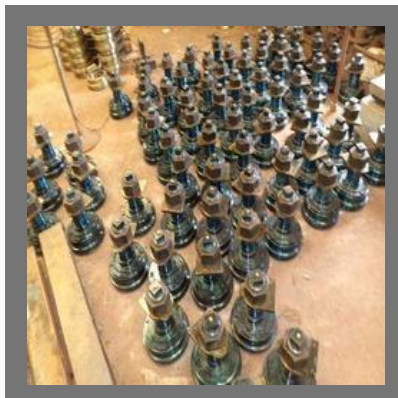
Guide Rollers
